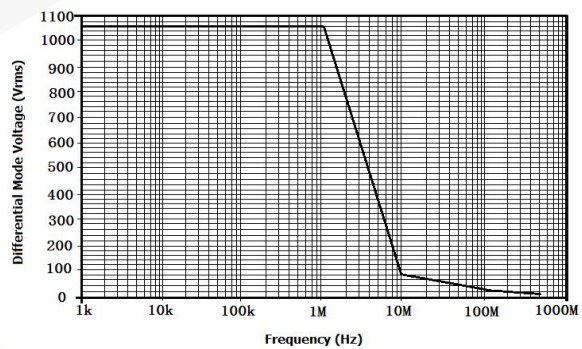
图 2 DP6150A 最大差模电压 VS 频率
