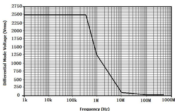
图 3 DP6350A 最大差模电压 VS 频率
