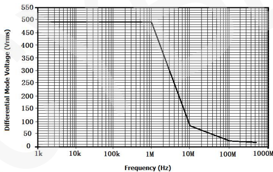
图 1 DP6070A 最大差模电压 VS 频率
