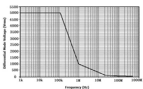
图 4 DP6700A 最大差模电压 VS 频率
